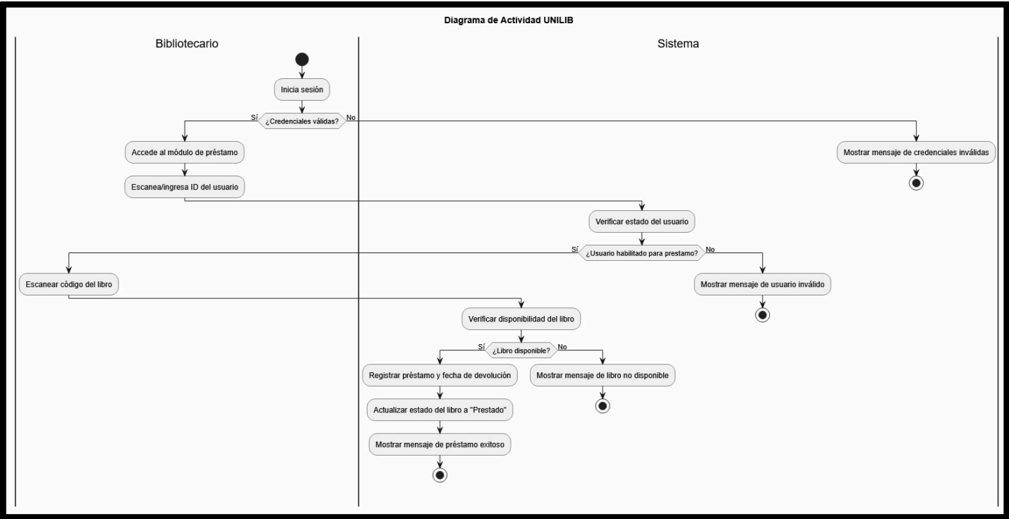
Diagrama de Actividad UNILIB
