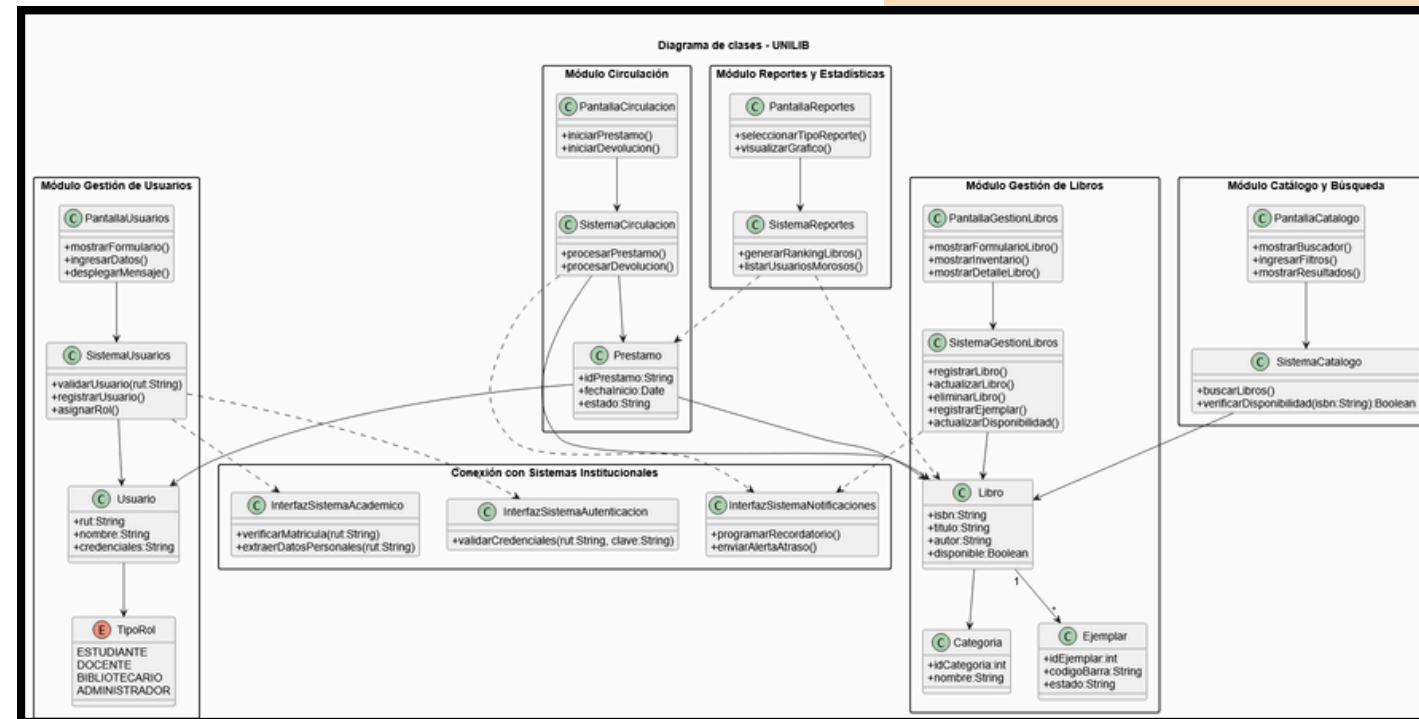
Diagrama de clases UNILIB
